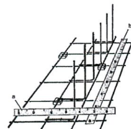
基礎配筋状況
