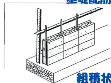
基礎配筋状況
